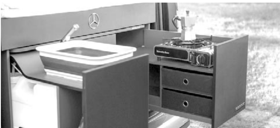
Mercedes-Benz T osztály, Marco Polo modul, a kivehető asztal
