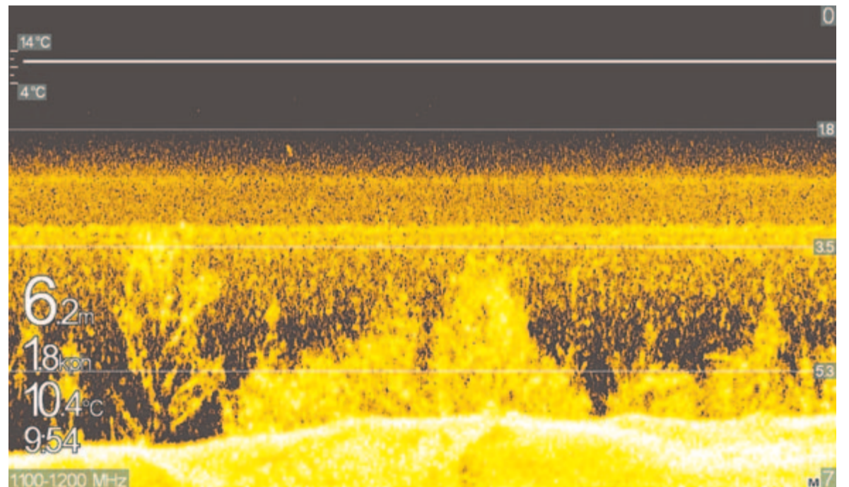
Erdő a Medve-tó mélyén, ahogy azt a hangradar által kirajzolt függőleges metszet mutatja. A 2-3 méter körüli vízszintes struktúra a haloklin réteget jelöli. A jobb oldali skála a mélységet jelöli. A szonárfelvételt dr. Hantz Péter készítette.
