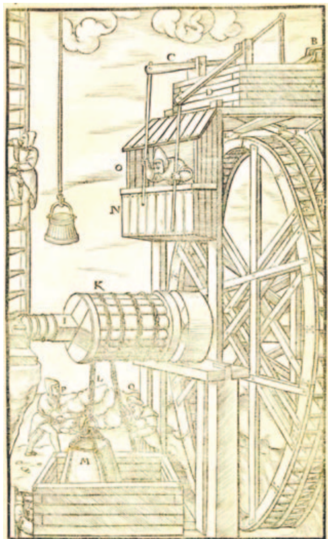
A Thurzó-féle merítómű Agricola De re metallica című művéből
