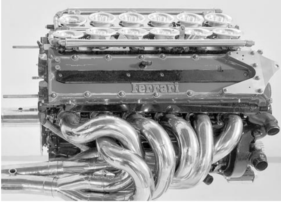
Ferrari V12-es motor
